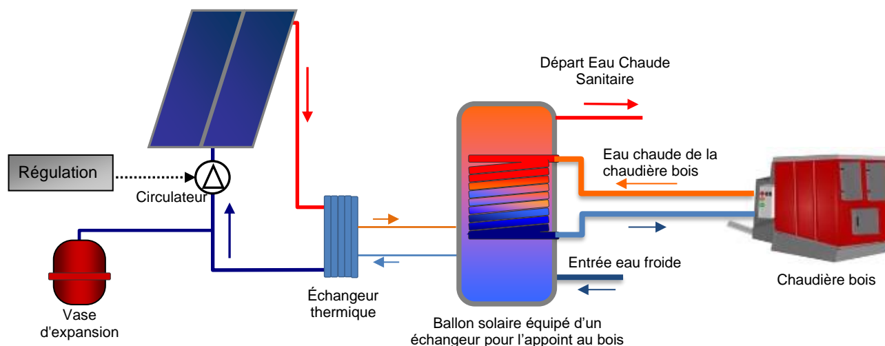
Schéma d'un Chauffe-Eau Solaire Collectif
